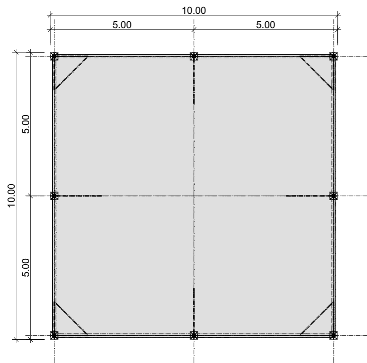
GRUNDRISS PAGODENZELT 10X10 METER
