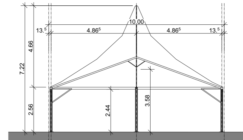
QUERSCHNITT PAGODENZELT 10X10 METER
