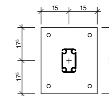
BODENPLATTE 30X35 CM
