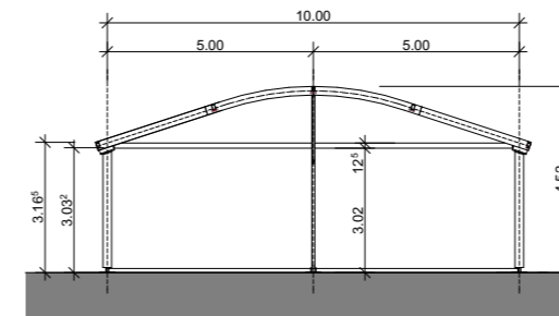
QUERSCHNITT ZELT 10 METER MIT BOGENDACH
