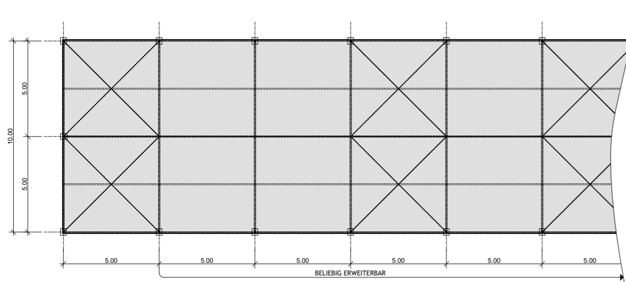
GRUNDRISS ZELT 10 METER MIT BOGENDACH
