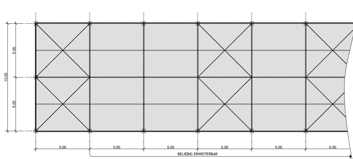
GRUNDRISS ZELT 10 METER
