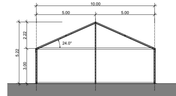
QUERSCHNITT ZELT 10 METER
