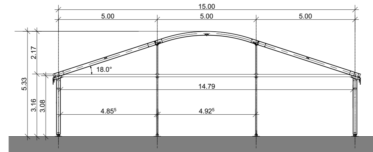
QUERSCHNITT ZELT 15 METER
