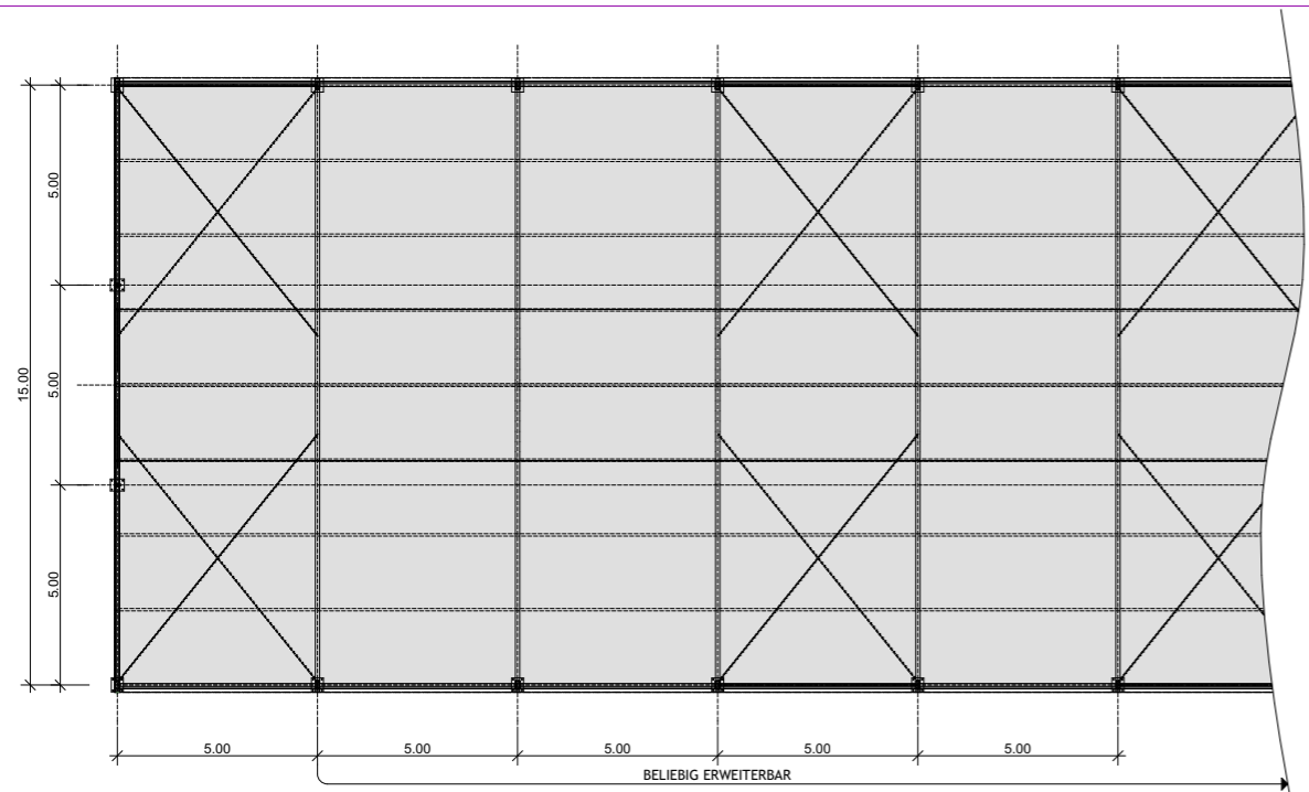
GRUNDRISS ZELT 15 METER
