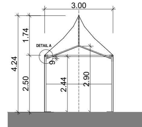
QUERSCHNITT PAGODENZELT 3X3 METER
