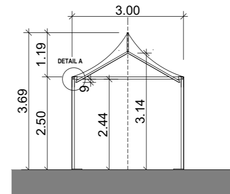
QUERSCHNITT PAGODENZELT 3X5 METER CITY
