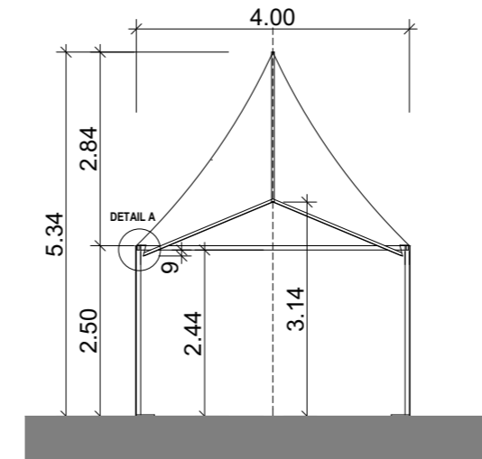
QUERSCHNITT PAGODENZELT 4X4 METER
