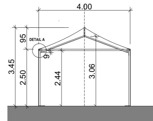
QUERSCHNITT PAGODENZELT 4X4 METER CITY
