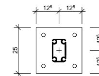
BODENPLATTE 25X25 CM
