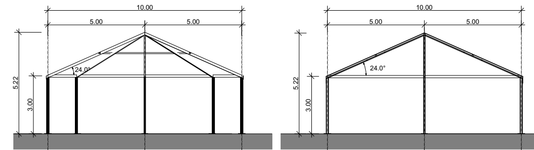
QUERSCHNITT ZELT 10 METER 8-ECK MIT VERLÄNGERUNG
