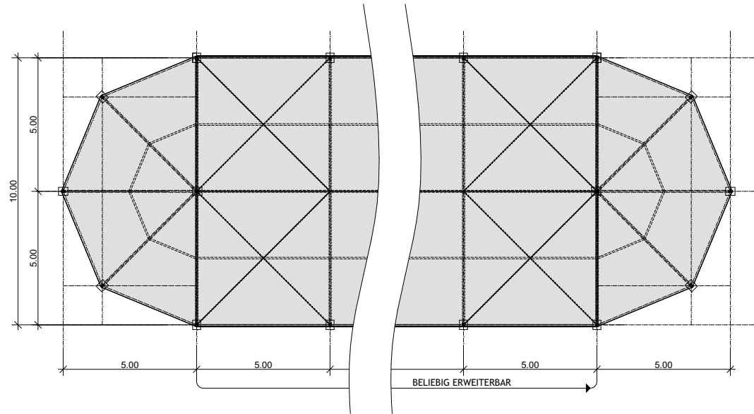
GRUNDRISS ZELT 10 METER 8-ECK MIT VERLÄNGERUNG
