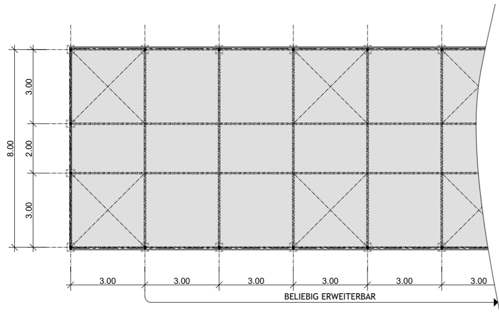
GRUNDRISS ZELT 8 METER
