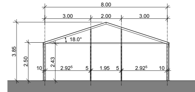
QUERSCHNITT ZELT 8 METER
