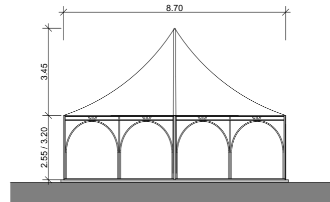
QUERSCHNITT CHAPITEAU 1-MASTER
