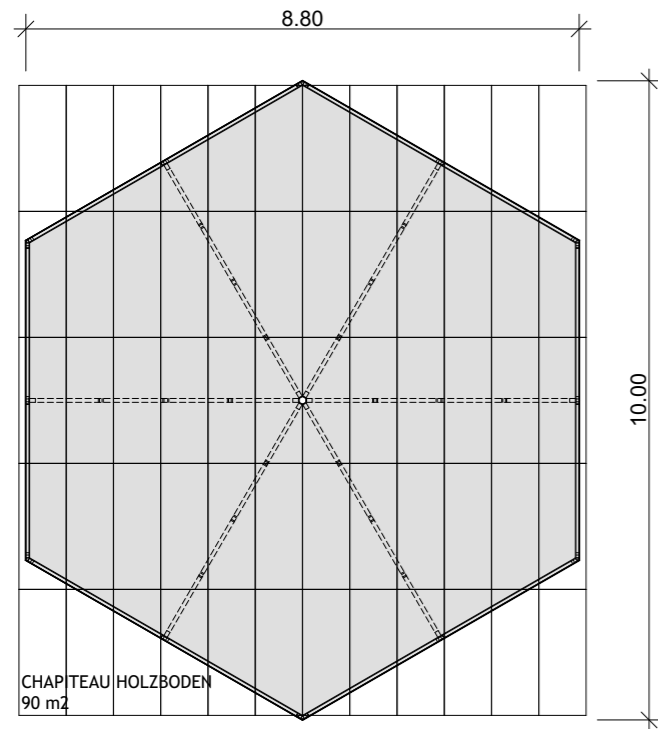
GRUNDRISS CHAPITEAU 1-MASTER
