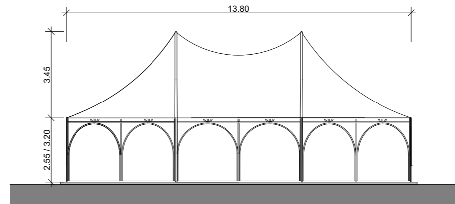
QUERSCHNITT CHAPITEAU 2-MASTER
