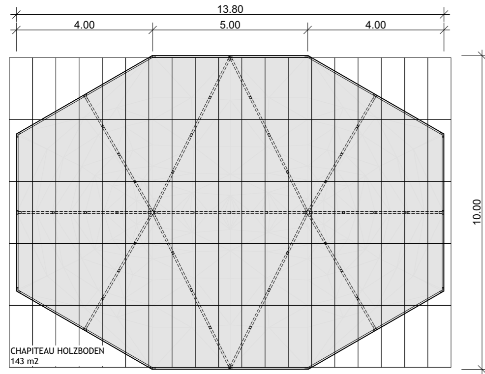
GRUNDRISS CHAPITEAU 2-MASTER
