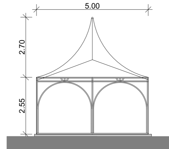
QUERSCHNITT CHAPITEAU PAGODE
